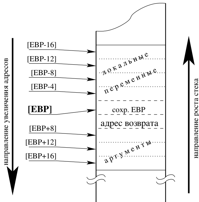
Рис. 3.5. Структура стекового фрейма
