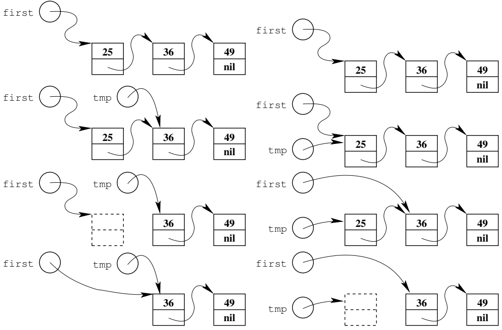
Рис. 2.9. Два способа удаления первого элемента односвязного списка
