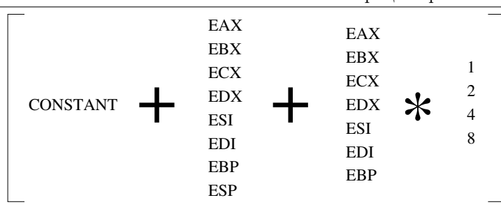
Рис. 3.2. Общий вид исполнительного адреса
