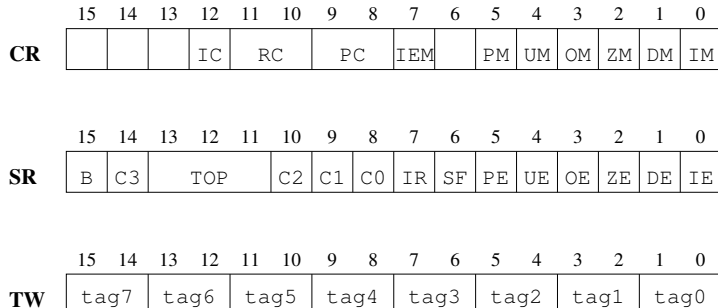
Рис. 3.11. Разряды регистров CR, SR и TW
