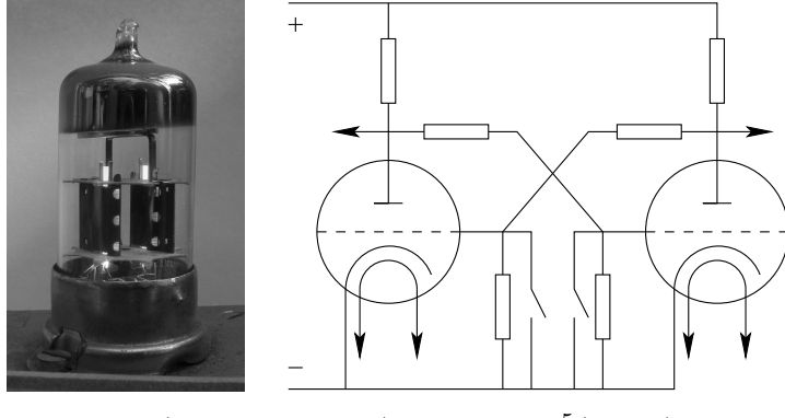
Рис. 1.1. Радиолампа (двойной триод) в действии 5 (слева); схема триггера на двух триодах (справа)
