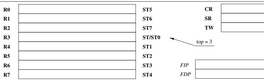
Рис. 3.10. Регистры арифметического сопроцессора
