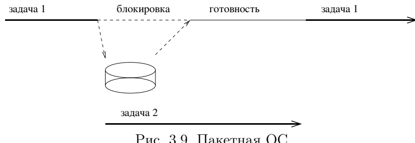
Рис. 3.9. Пакетная ОС
