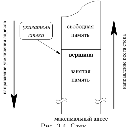
Рис. 3.4. Стек
